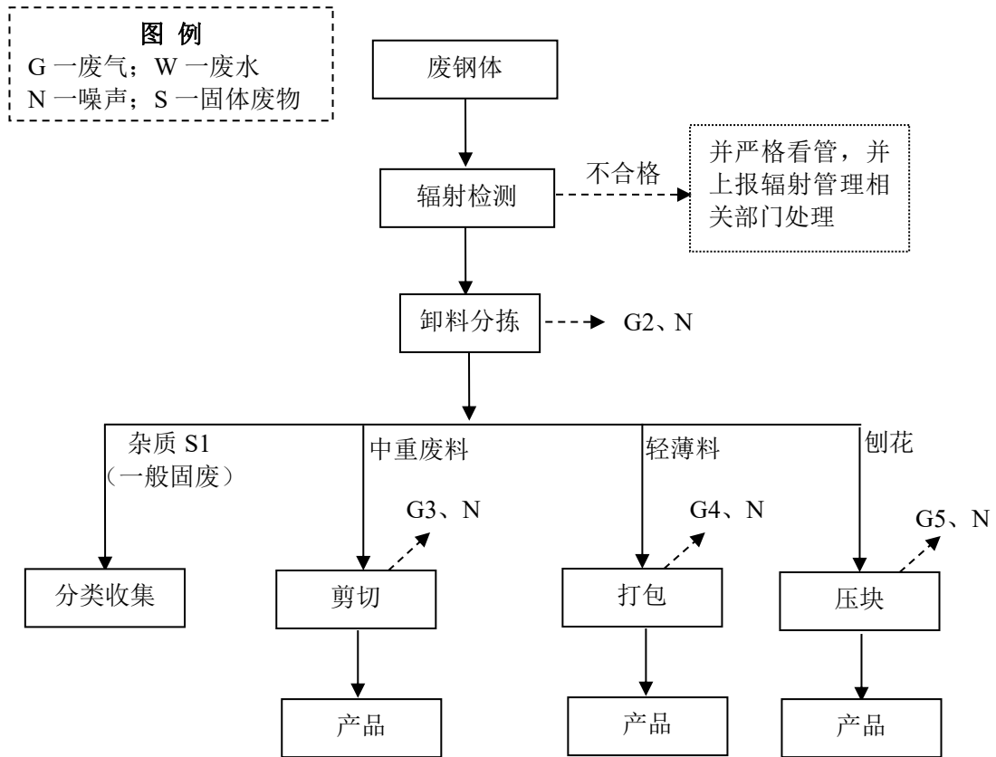
图 2-3 项目运营期生产工艺流程及产污环节
