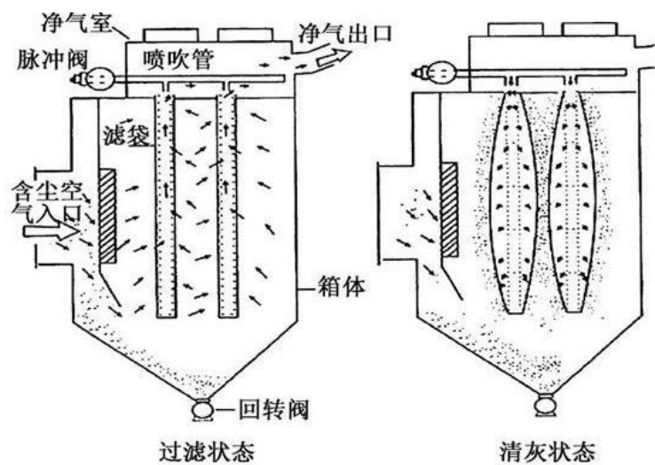
图4-1 布袋除尘器工艺流程示意图
